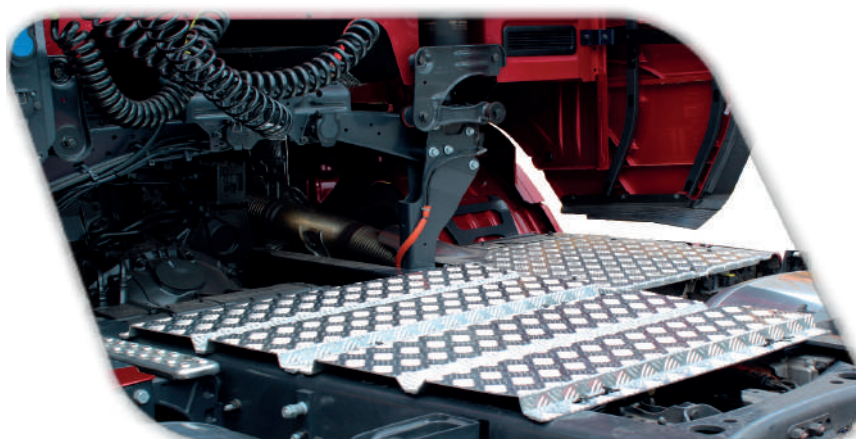
Plataforma V-790 aplicada
