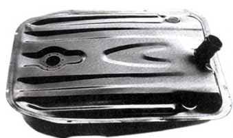
D-613 - 57 Litros (N° Compatível: BD3M9002A) Com Retorno Bocal Reto Boia 6 Parafusos Compatível com Ford Corcel I 1971...1977 Medidas: 775(comprimento) x 600(largura) x 200(altura)mm
