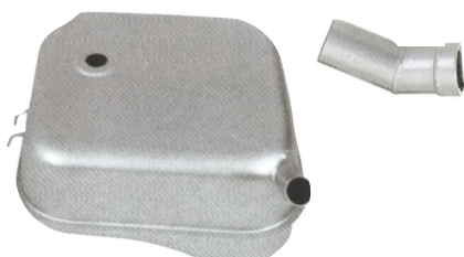
Compatível com Toyota Bandeirante 1970...1992 D-614 - 48 Litros Medidas: 550 (comprimento) x 480 (Largura) x 290 (altura)mm Nº Compatível: 97610255 D-614D - Bocal de Abastecimento
