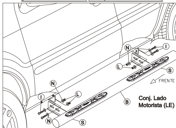
Fixação suporte dianteiro lado motorista.
