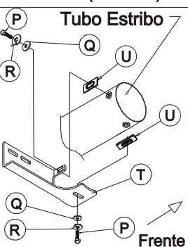
Fixação suporte dianteiro lado motorista.
