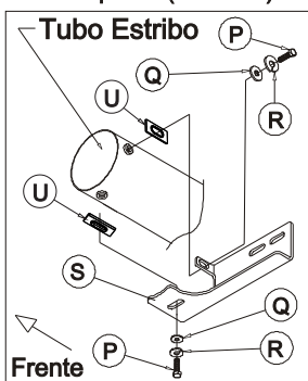
Fixação suporte traseiro lado motorista.
