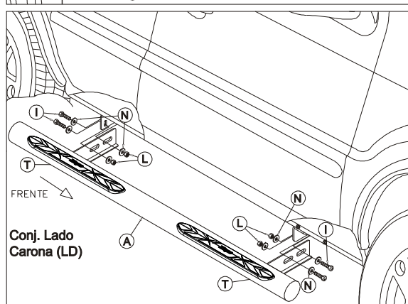
Fixação suporte dianteiro lado carona.
