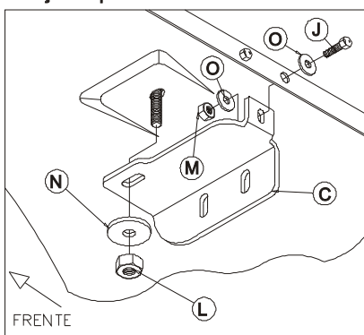
Fixação suporte dianteiro lado carona.
